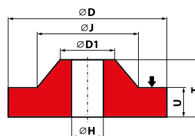
3802 - D/J × T/U × H - ... - V - Zeichnung Nr.
