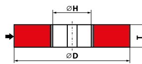
101X - D × T × H - Zeichnung Nr.
