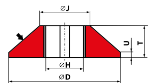
301X - D/J × T/U × H - Zeichnung Nr.
