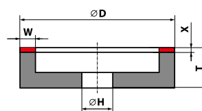
6A2 - D × T-X × W × X × H
