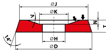
2001 - D/J × T × H - ... - V - Zeichnung Nr.
