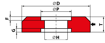
7X - D × T × H - P...F...G... - Zeichnung Nr.
