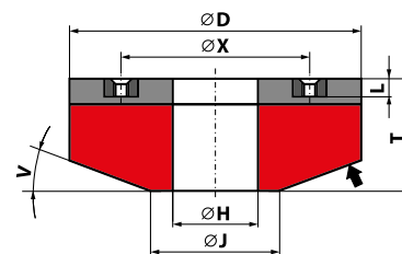
3611 - D x T x H - ... - V - Zeichnung Nr.
